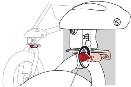
Bouton de réglage de l'alignement
